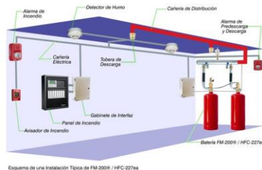
Esquema de una Instalación Típica de FM 200B / HFC 227ea
